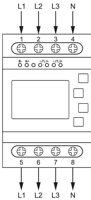
3P4W
