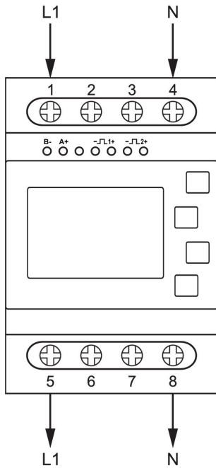
1P2W(L+N)
