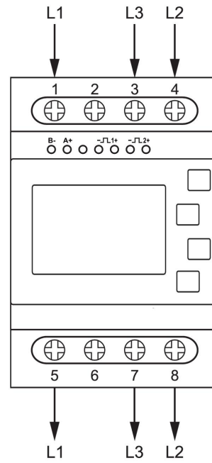
3P3W
